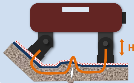
Magnetización Magnetisation
